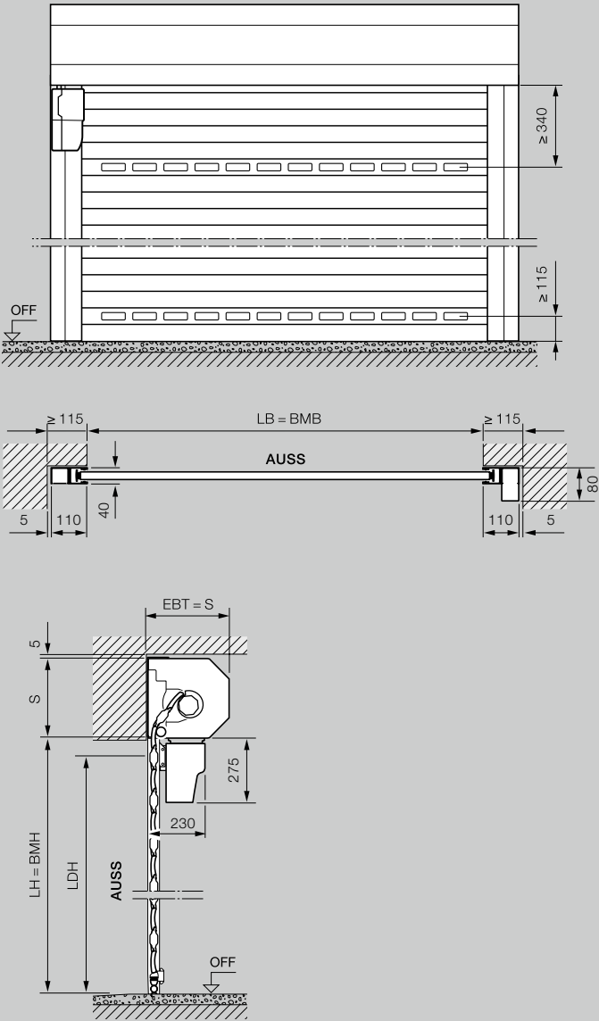
Storleksområde in- och utvändig rullport
