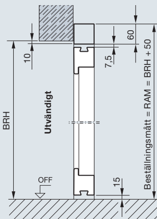
Vertikalsnitt Exempel: montage bakom öppningen
