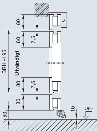
Horizontalsnitt Skjutport ST 500 med gångdörr
