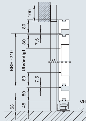
Vertikalsnitt Skjutport ST 500 med gångdörr
