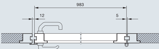
Horizontalsnitt Vippport ET 500 med gångdörr
