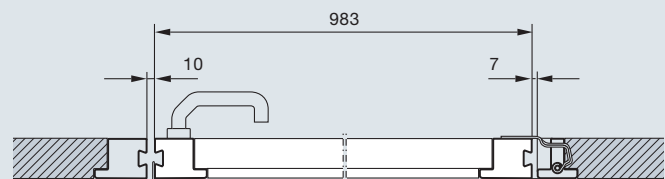
Horizontalsnitt Skjutport ST 500 med gångdörr
