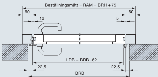
Horizontalsnitt Montage bakom öppningen
