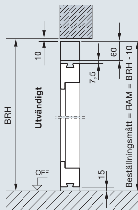
Vertikalsnitt Exempel: montage i öppningen
